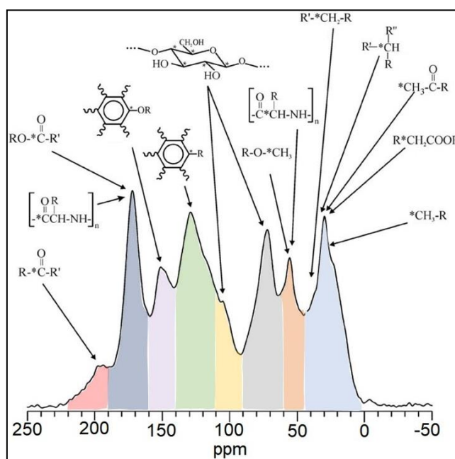
Figura 3. Espectro representativo 13 C NMR CP/MAS de AH isolados de solos isolado de Uncompahgre (tomado e modificado de Keeler et al. 2006) 44
