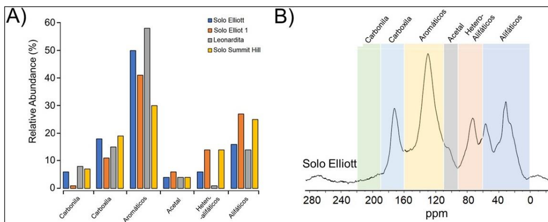
Figura 2. Quantidades relativas de estruturas de AH nas SH que propõe a SISH como padrões (A). Espectro 13 C NMR CP/MAS de AH de solo Elliott mostrado como padrão na SISH (tomado e modificado das informações disponíveis no site oficial da SISH, https://humic-substances.org ). 43 Solo Elliott: solo fértil presente no estado de Illinois, USA. Solo Summit Hill: solo coletado de Port Hill, Nova Zelanda
