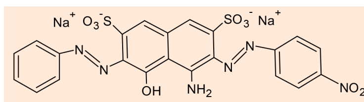
Figura 1. Estrutura do corante preto de amido 10 B
