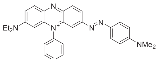
Janus Green B
